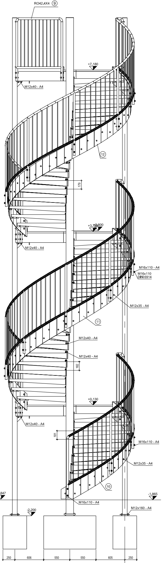
Vorderansicht M1:20
