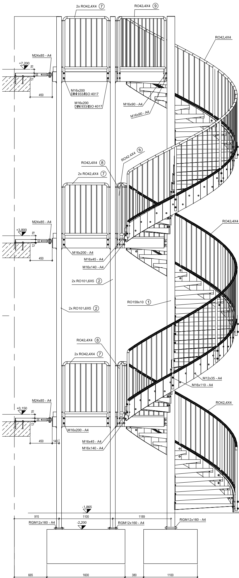
Seitenansicht M1:20
