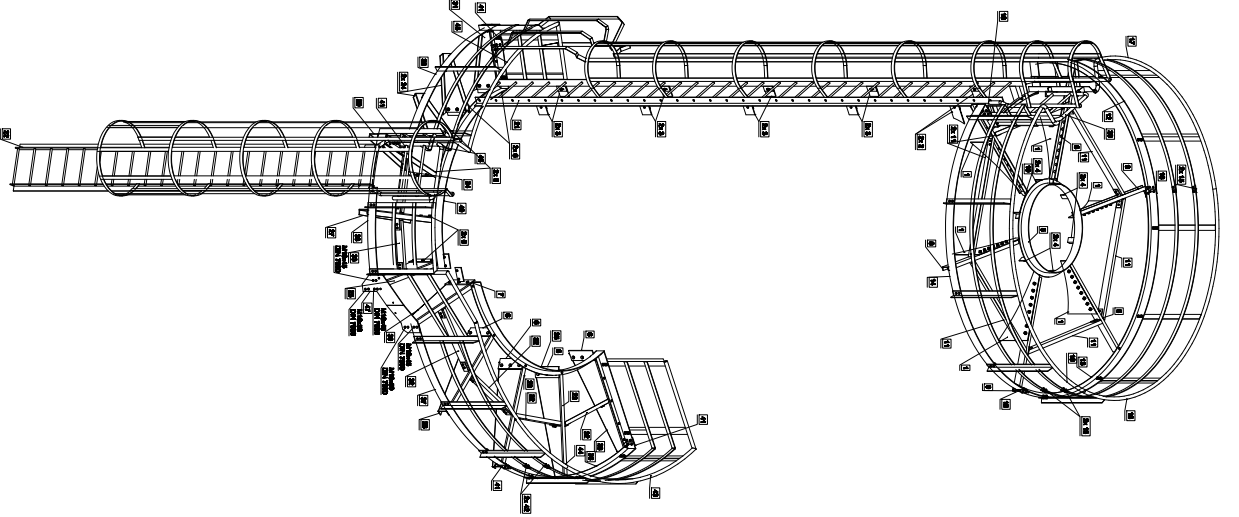
Übersicht ohne Geländer und Säulen, M1:20
